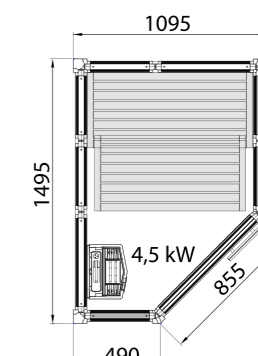
IMPRESSION SAUNA i1115/C
