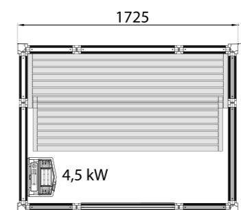
IMPRESSION SAUNA i1713
